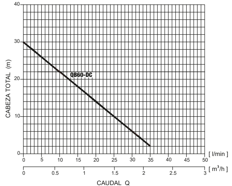
Imagen 4. Curva de operación de la bomba
